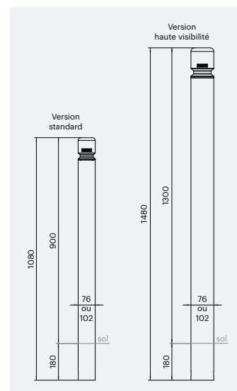
Système d'amovibilité pour potelets Serrubloc® 21
